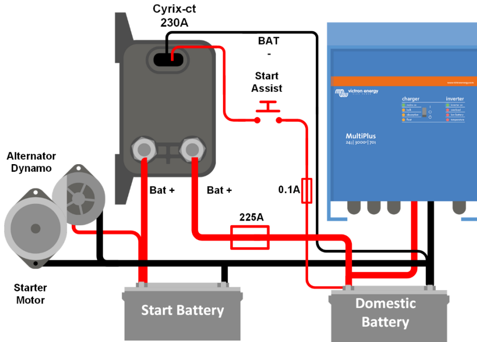
Cyrix-ct 12/24-230: bağlantı diyagramı
